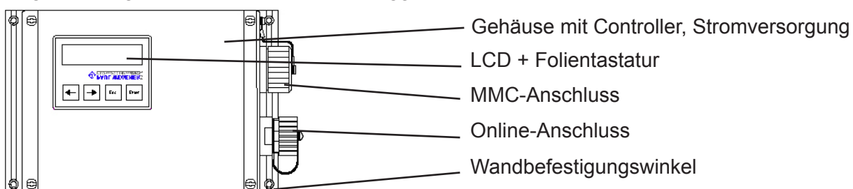
Bild 1 Ausführung N6/7
